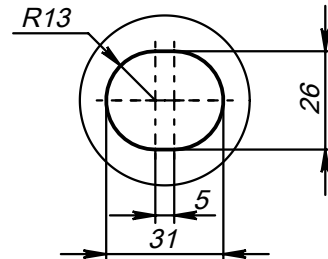
A (1 : 2)
