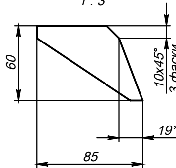
Поз.4 (Косынка) 1 : 3
