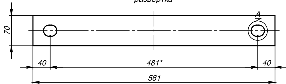
Поз.1 (Полухомут) развертка
