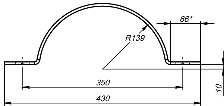
Поз.1 (Полухомут)
